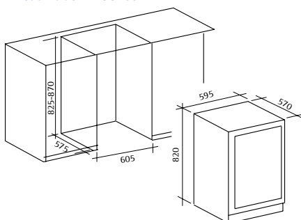
Einbaumaße WKU820S
