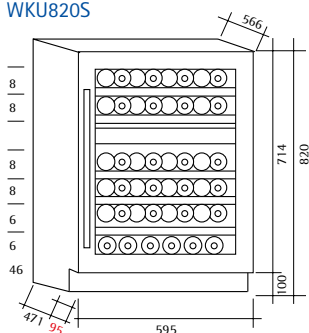
Einbaumaße WKU820S
