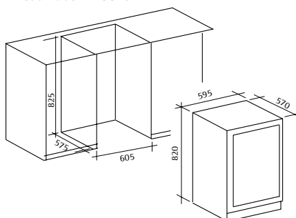
Einbaumaße WKU820
