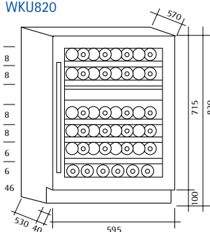
Einbaumaße WKU820
